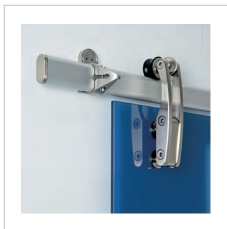
■ SISTEMA TECNICO DI SCORRIMENTO CON BINARIO IN ALLUMINIO ANODIZZATO E PINZE SORREGGI VETRO IN ACCIAIO INOX (ART NS/1/13)
